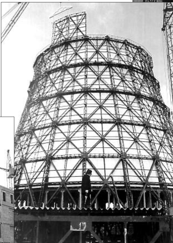
Градирня № 3 ТЭЦ-5.
