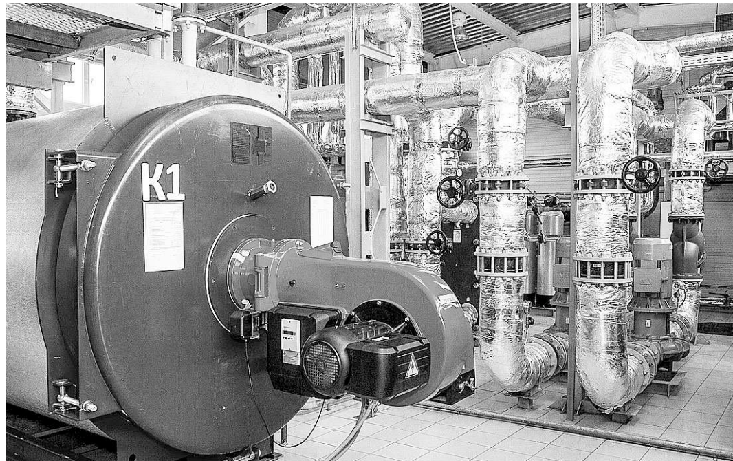
Колыванская газовая котельная, одна из самых современных в области, — успешный пример государственно-частного партнёрства.
