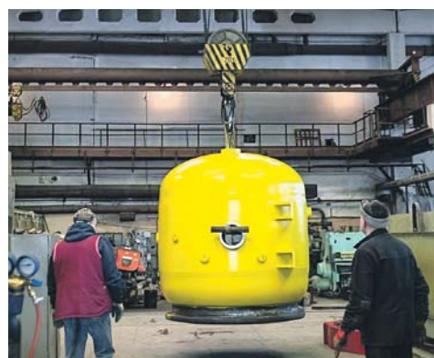
Эта камера способна выдержать взрыв, который уничтожит грузовой автомобиль.
