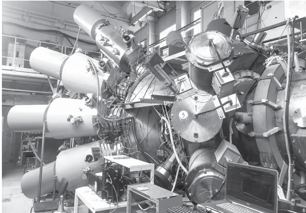
Через зелёные и оранжевые «бочки» по краям ГДМЛ в центр установки влетают пучки нейтральных атомов, сталкиваясь с плазмой.
