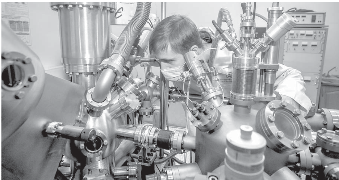
Фотоэлектронный спектрометр в Институте катализа СО РАН помогает учёным в разработке катализаторов. 2021 год.
