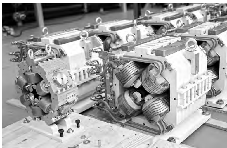
Задача квадрупольных магнитов — фокусировка летящего по кольцу бустера пучка электронов.
