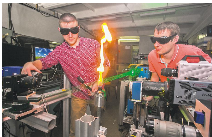
Лазерные измерения в лаборатории термохимической аэродинамики новосибирского Института теплофизики имени С. С. Кутателадзе.
