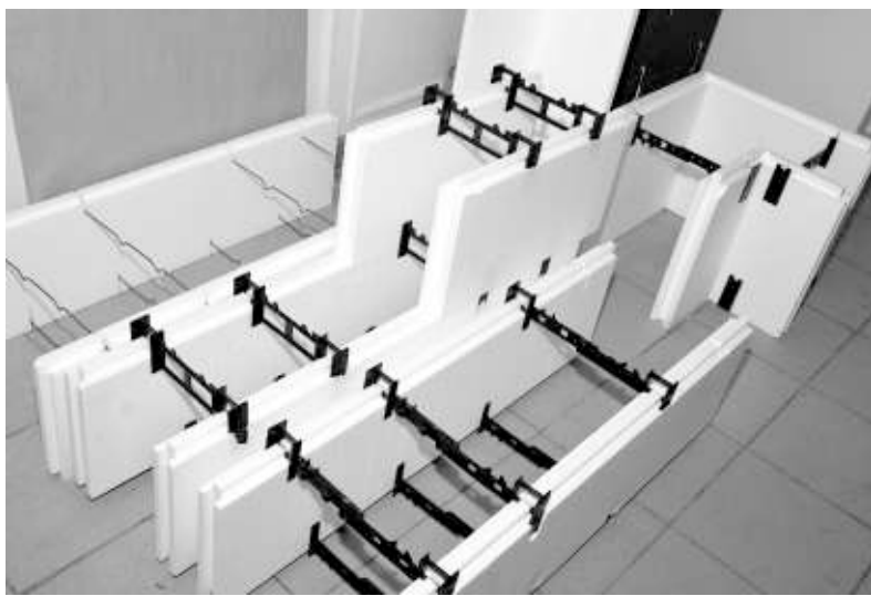
Несъёмная опалубка — конструктор из пенополистирольных блоков, которые стыкуются между собой с помощью пазовых креплений.
